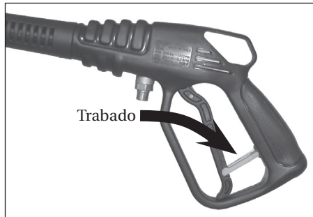
Figura 14 - Gatillo trabado
