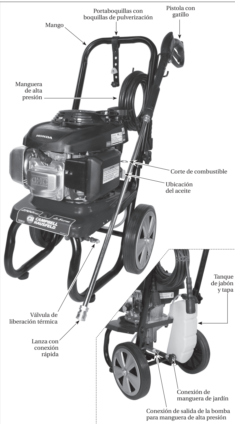
Figura 7 - Componentes de la lavadora a presión
