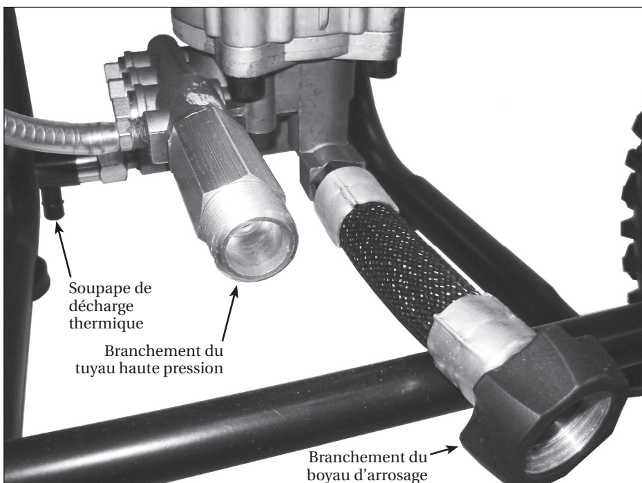
Figure 9 - Branchements de la pompe
