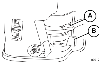
Figura 3-2. Válvula de combustible y cebador
