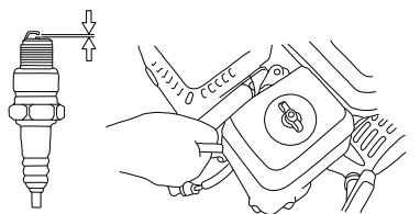
Figura 4-8. Bujía
