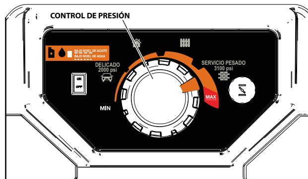
Figura 19 - Cuadrante de potencia
