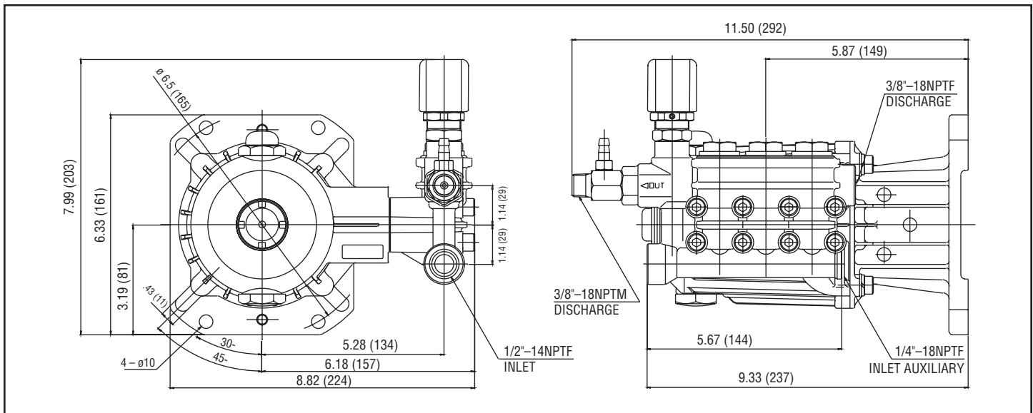
Model 67PPX39G11
